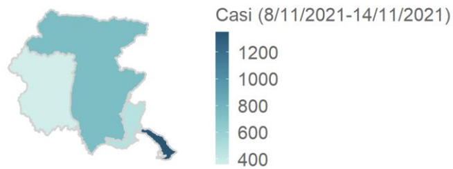
Friuli-Venezia Giulia 2907 casi
