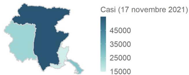
Friuli-Venezia Giulia 120594 casi
