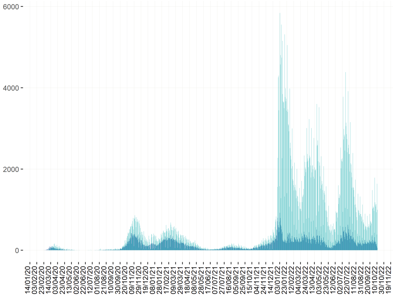
Curva epidemica
